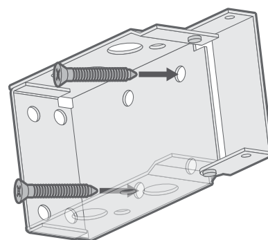
Zijkantmontage
